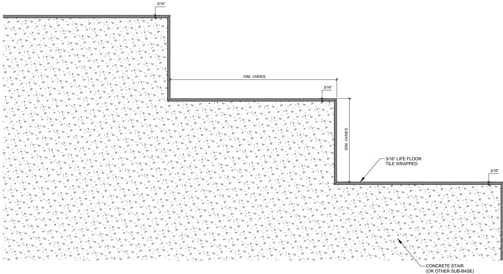
1 LIFE FLOOR STAIR WRAP VARIANT 2 SCALE: 3" = 1'-0"
